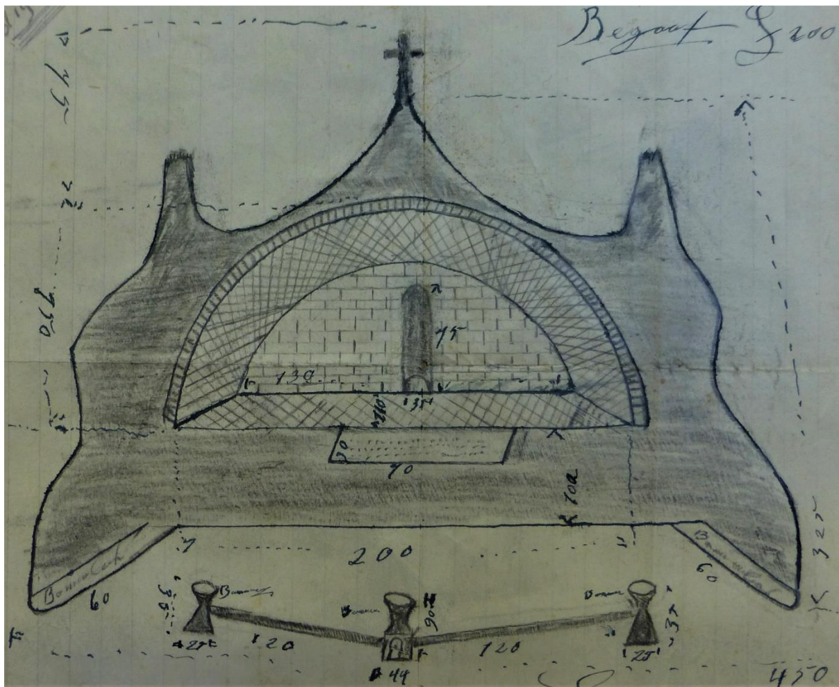
Ontwerp van de Baarschotse Grot in 1946 aan de verdwenen Vestweg naar het Gijseleind
